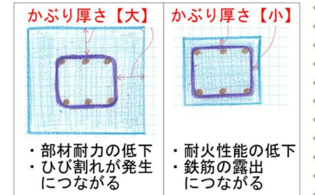
★かぶり厚さの違いによる比較★
