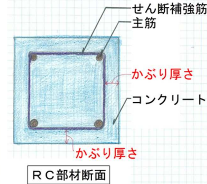
★かぶり厚さの説明★
